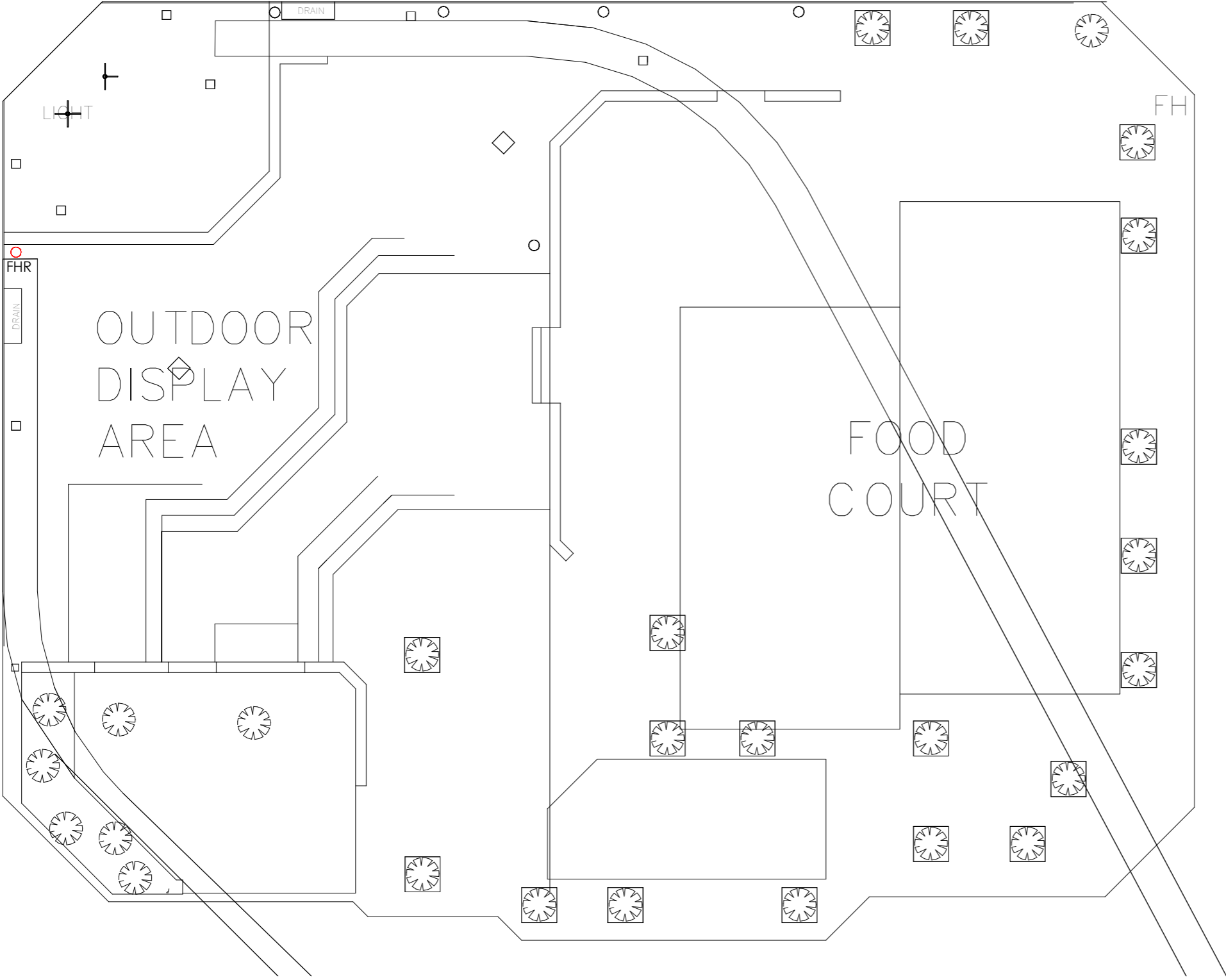
1 STAND LAYOUT 1 : 7000
