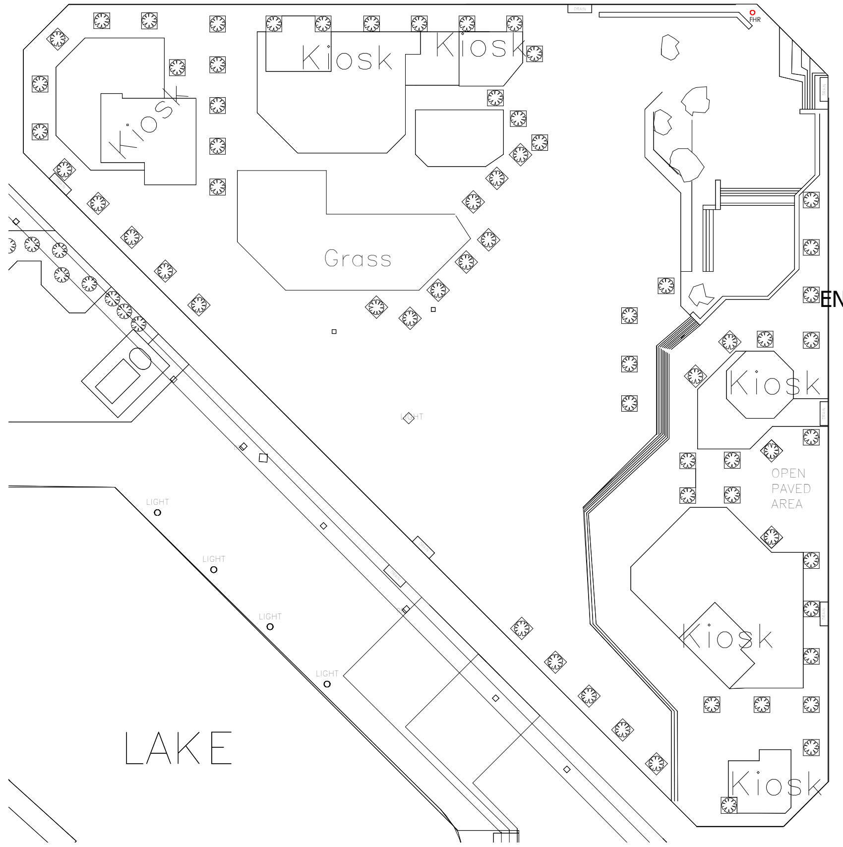
1 STAND LAYOUT 1 : 12001
